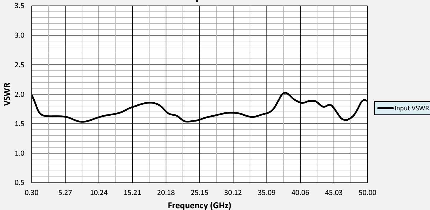
Input VSWR
