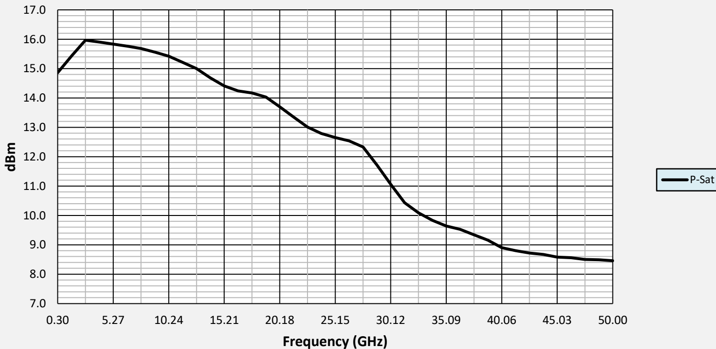
P-Sat
